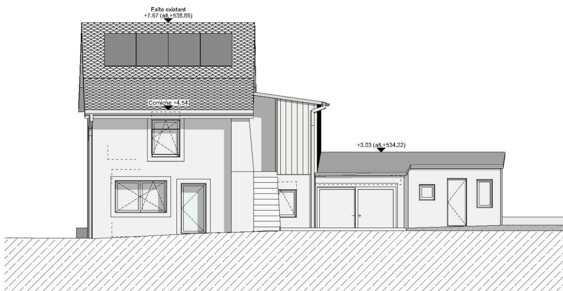
Elévation sud-ouest
